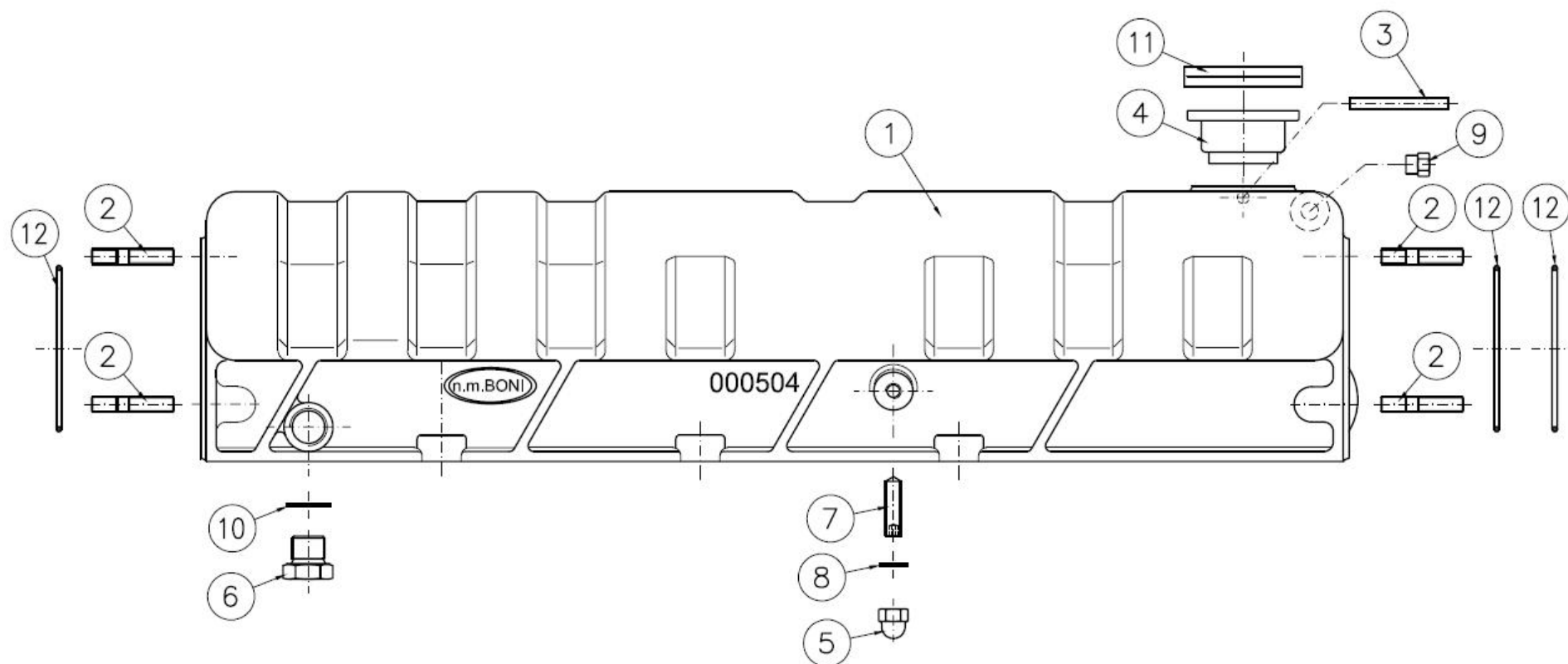
CORPO SCAMBIATORE DI CALORE PER MOTORE BV 4404 AN – TS – TSI CODICE 00.90.61-3
