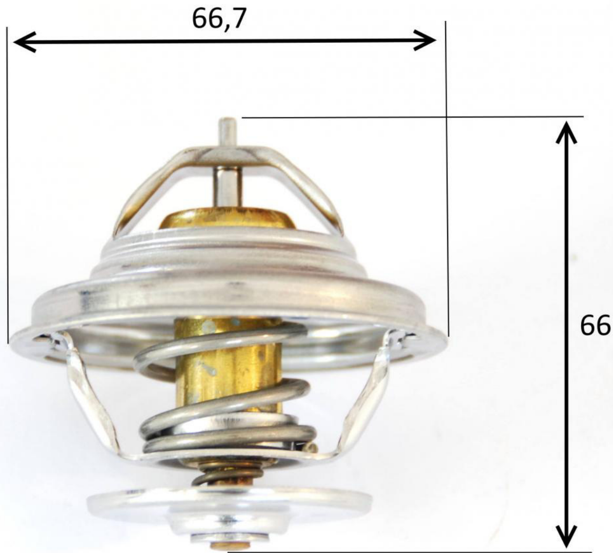
VALVOLA TERMOSTATICA codice: 00.98.66
